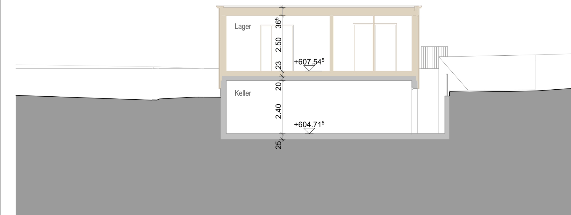
Längsschnitt B
