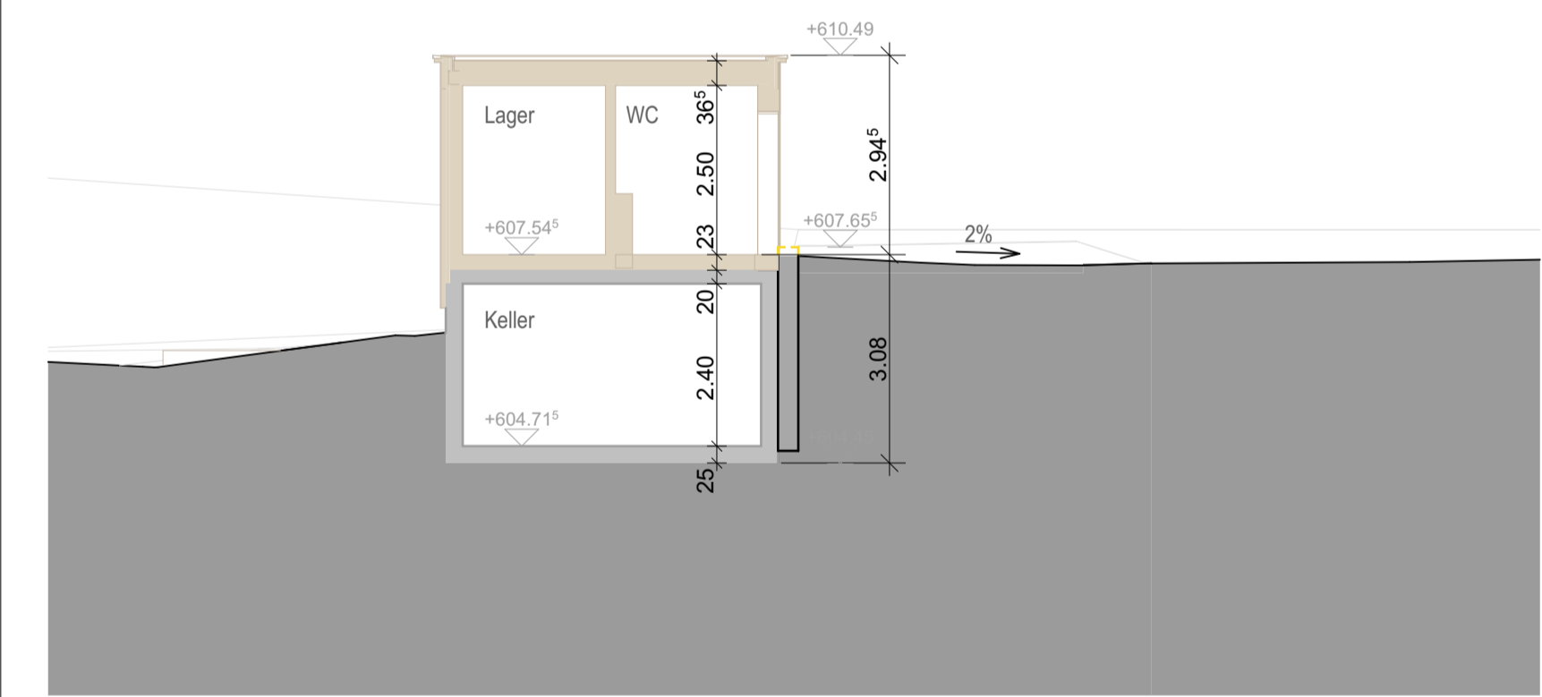
Querschnitt A
